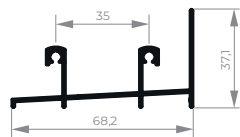
EXL-055 Terminal da persiana 0,352 kg/m
