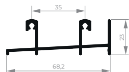
EXL-260 Trilho de correr inferior 2 planos 0,555 kg/m
