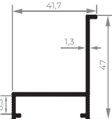
RA-042 Arremate 0,252 kg/m
