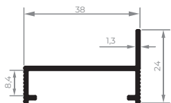
CA-060 Contramarco 0,254 kg/m
