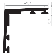
RA-013 Arremate de piso 0,243 kg/m
