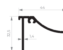
EXL-169 Arremate de piso 0,353 kg/m
