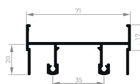
EXL-001 Trilho de correr superior 2 planos 0,773 kg/m
