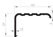
RA-013 Arremate de piso 0,243 kg/m
