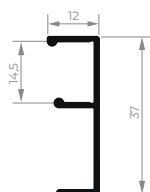
RA-88347 Arremate 0,186 kg/m
