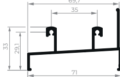
EXL-002 Trilho de correr inferior 2 planos 0,688 kg/m
