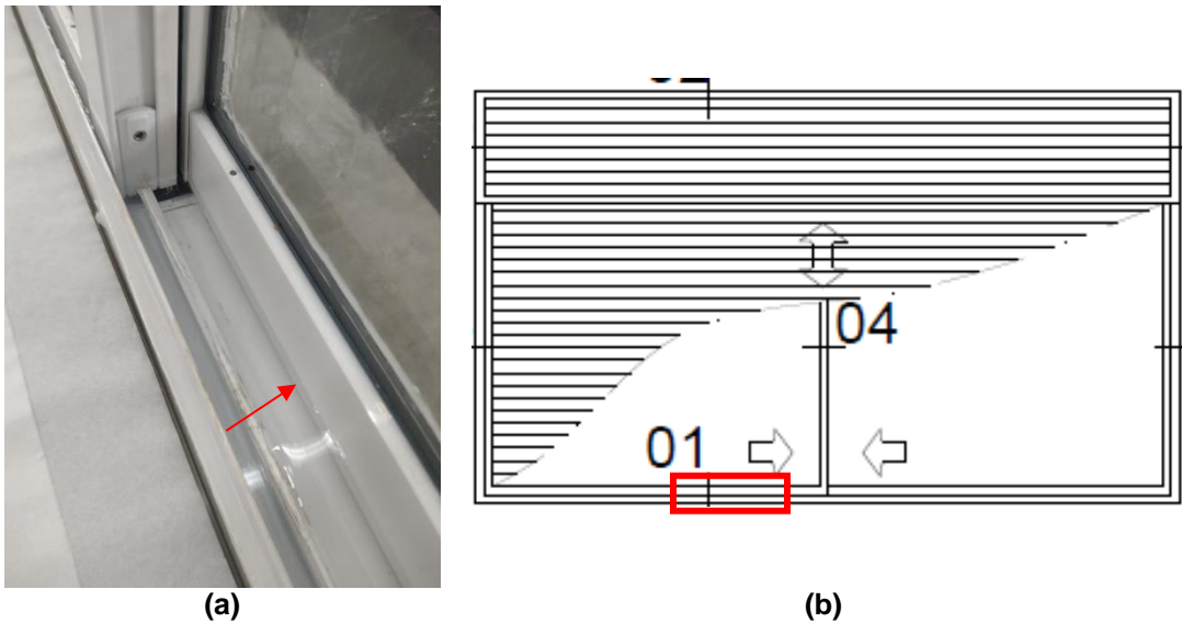
Figura 5 – (a) Indicação da presença de água no trilho, e (b) localização do ponto da ocorrência
