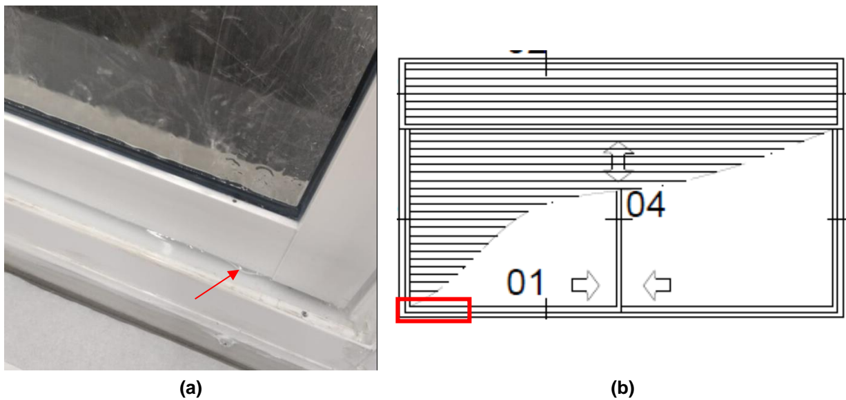
Figura 6 – (a) Indicação da ocorrência de PI, e (b) localização do ponto de PI
