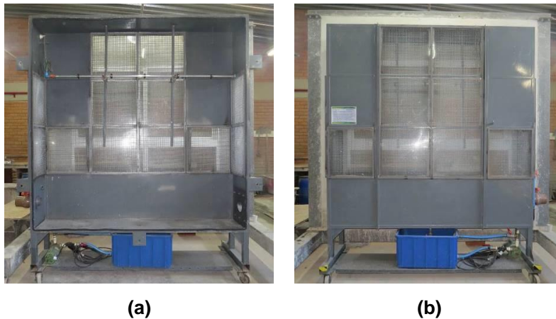
Figura 2 – Vistas da câmara de ensaio: (a) vista interna, e (b) vista externa
