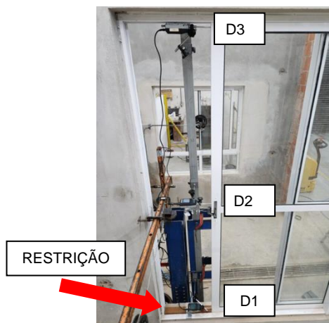
Figura 2 – Instrumentação de ensaio de resistência horizontal com um canto imobilizado
