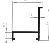
CA-098 Contramarco 0,356 Kg/m
