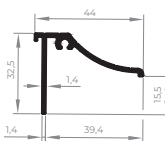
EXL-169 Arremate 0,353 Kg/m
