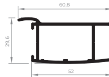
EXL-336 Marco lateral integrada 3 planos 0,765 Kg/m
