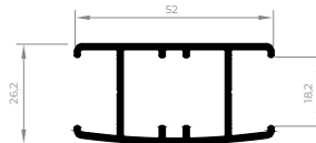
ALV-2023 Montante central veneziana 0,580 Kg/m
