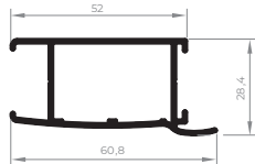
ALV-2010 Travessa superior inferior veneziana janela 0,633 Kg/m
