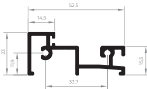
ALV-20902 Trilho inferior acople 0,613 Kg/m
