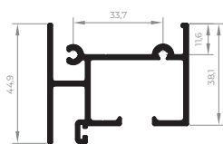
ALV-20901 Trilho superior acople 0,900 Kg/m
