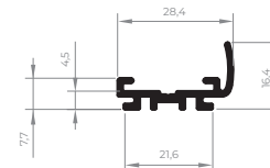
ALV-20994 Perfil de reversão veneziana 0,253 Kg/m
