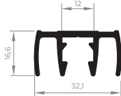
ALV-2006 Matajunta lateral 0,382 Kg/m
