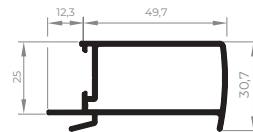
ALV-2018 Montante central interno da folha 0,626 Kg/m
