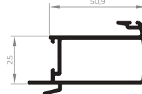
ALV-2027 Montante intermediário da folha 60 0,730 Kg/m
