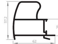
ALV-2016 Montante bi-tubular central interno da folha 0,911 Kg/m
