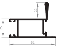
ALV-2014 Montante central da folha 0,842 Kg/m
