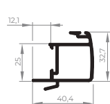
EXL-503 Montante central intermediário da folha 0,549 Kg/m
