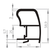
EXL-400 Montante bi-tubular central interno reforçado 1,038 Kg/m
