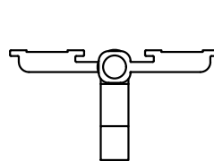
DETALHE DE APLICAÇÃO DA DOBRADIÇA SEM PUXADOR: (escala 1:1)
