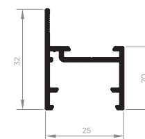
EXL-088 Marco perimetral fixo 0,278 Kg/m
