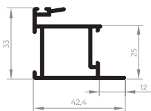
EXL-1250 Perfil montante lateral folha 1,185 Kg/m
