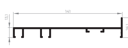
EXL-123 Montante lateral de correr 4 planos 0,871 Kg/m
