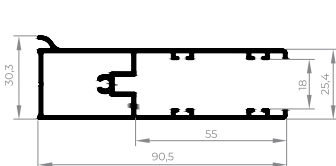
EXL-800 Perfil trilho persiana 55 mm 1,044 Kg/m
