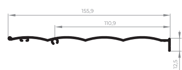
EXL-516 Tampa externa janela integrada 0,698 Kg/m
