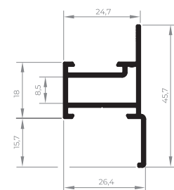
EXL-276 Pingadeira do marco maxim-ar 0,176 Kg/m
