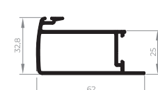
ALV-2015 Montante central externo da folha 0,690 Kg/m
