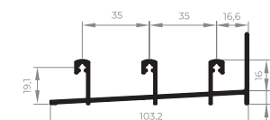
EXL-230 Trilho de correr inferior porta 3 planos 0,930 Kg/m
