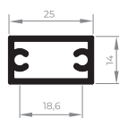
ALV-20706 Tubo retangular com olhal 0,313 Kg/m
