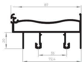
EXL-507 Marco intermediário integrada tubular 1,331 Kg/m
