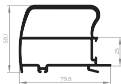
EXL-250 Montante central da folha 0,796 Kg/m
