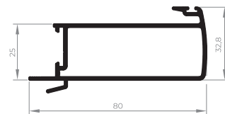
EXL-245 Montante lateral da folha 0,623 Kg/m
