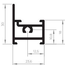
EXL-082 Travessa superior maxim-ar 90° 0,382 Kg/m
