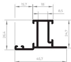
EXL-200 Montante com escova maxim-ar 0,402 Kg/m
