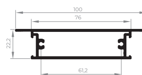
EXL-666 Travessa inferior porta 0,974 Kg/m
