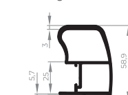
EXL-400 Montante bi-tubular central interno reforçado 1,038 Kg/m
