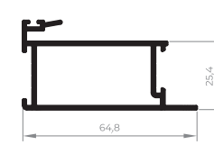
EXL-227 Travessa intermediária da folha 0,556 Kg/m
