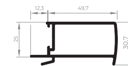
ALV-2018 Montante central interno da folha 0,626 Kg/m
