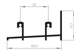
EXL-228 Trilho de correr inferior 2 planos 0,600 Kg/m
