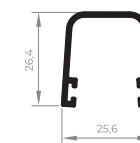
EXL-107 Vedação do montante 0,272 Kg/m
