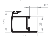
EXL-502 Montante central externo da folha 0,512 Kg/m
