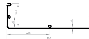
EXL-032 Tampa interna janela integrada 1,494 Kg/m
