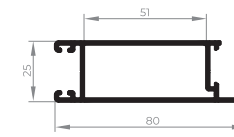
ALV-2082 Montante lateral da folha 0,803 Kg/m
