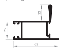
ALV-2014 Montante central da folha 0,842 Kg/m
