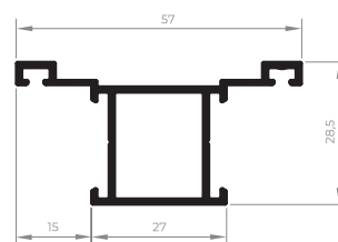
EXL-085 Travessa vertical sem olhal maxim-ar 0,491 Kg/m
