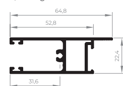
EXL-246 Travessa inferior da folha 0,645 Kg/m
