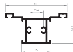
EXL-086 Travessa vertical com olhal maxim-ar 0,574 Kg/m
