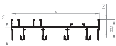
EXL-121 Trilho de correr superior 4 planos 1,577 Kg/m
