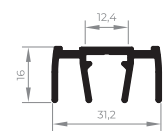
EXL-291 Matajunta lateral 0,358 Kg/m
