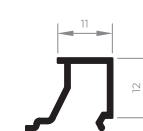
EXL-102 Baguete 0,102 Kg/m
