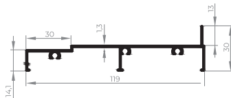
EXL-802 Marco inferior integrada c/ peitoril 0,757 Kg/m
