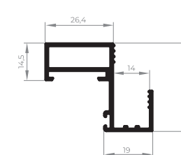
AFV-007 Folha encaixilhada 0,542 Kg/m
