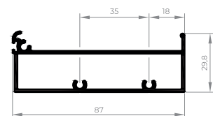
AFV-004 Marco intermediário tubular liso 1,085 Kg/m
