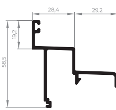
AFV-006 Batente inferior 0,676 Kg/m
