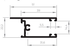
EXL-053 Travessa da folha 0,447 Kg/m
