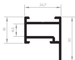
EXL-200 Montante com escova maxim-ar 0,402 Kg/m
