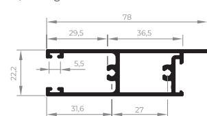
EXL-224 Travessa inferior da folha 0,790 Kg/m
