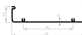
EXL-031 Tampa interna janela integrada 0,941 Kg/m
