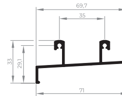
EXL-002 Trilho de correr inferior 2 planos 0,656 Kg/m
