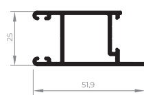
EXL-500 Montante lateral da folha 0,528 Kg/m
