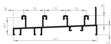
EXL-122 Trilho de correr inferior 4 planos 1,496 Kg/m
