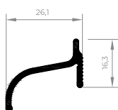
EXL-008 Veda vento trilho 0,219 Kg/m
