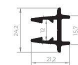
EXL-506 Matajunta central da folha 0,298 Kg/m
