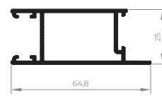
EXL-1505 Perfil montante central int. Folha 1,155 Kg/m
