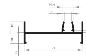
EXL-003 Marco lateral de correr 2 planos 0,517 Kg/m
