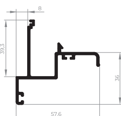
AFV-005 Batente superior 0,724 Kg/m
