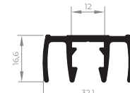
ALV-2006 Matajunta lateral 0,382 Kg/m
