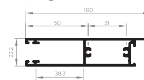
EXL-666 Travessa inferior porta 0,974 Kg/m
