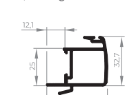
EXL-503 Montante central intermediário da folha 0,549 Kg/m
