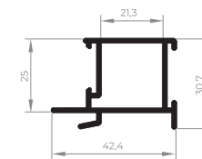
EXL-242 Montante central externo 0,623 Kg/m
