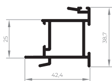
EXL-1502 Perfil montante central ext. Folha 0,593 Kg/m
