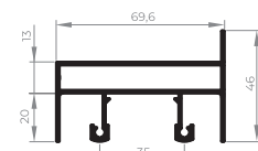
EXL-005 Trilho intermediário superior 1,107 Kg/m
