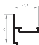
AFV-006 Batente inferior 0,676 Kg/m
