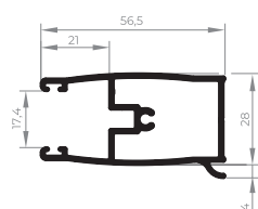
EXL-334 Marco Superior Integrada 3 planos 0,999 Kg/m
