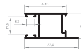
EXL-039 Montante da folha 0,516 Kg/m
