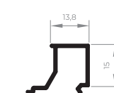
EXL-103 Baguete para Marco 0,126 Kg/m
