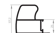
ALV-2016 Montante bi-tubular central interno da folha 0,911 Kg/m
