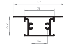
EXL-506 Matajunta central da folha 0,298 Kg/m
