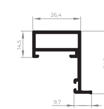
AFV-008 Folha colada 0,396 Kg/m
