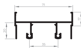
EXL-001 Trilho de correr superior 2 planos 0,773 Kg/m
