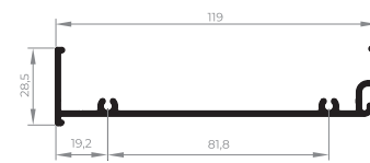
EXL-508 Marco superior integrada 0,794 Kg/m
