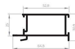
EXL-050 Perfil montante central ext. Folha 0,923 Kg/m
