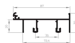
EXL-509 Marco intermediário integrada 0,802 Kg/m
