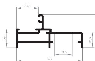
ALV-20708 Marco com suporte grade 0,711 Kg/m
