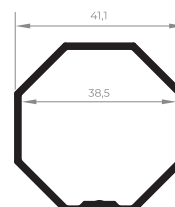
EXL-410 Tubo octogonal 40 mm 0,466 Kg/m
