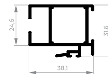
CEL-245 Montante lateral da folha 0,668 kg/m
