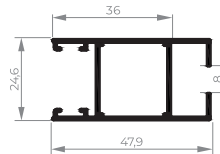
CEL-039 Montante da folha 0,545 kg/m
