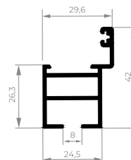
CEL-200 Montante maxim-ar com escova 0,478 kg/m
