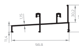
CEL-510 Trilho inferior integrada 0,775 kg/m
