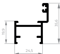
CEL-079 Travessa da folha 0,353 kg/m
