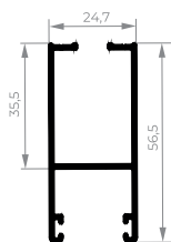
CEL-514 Guia para persiana 0,519 kg/m
