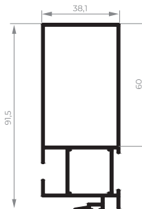
CEL-060 Montante central da folha com reforço 1,025 kg/m
