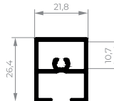
CEL-082 Travessa inferior maxim-ar 0,380 kg/m
