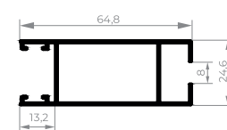
CEL-245 Montante lateral da folha 0,668 kg/m
