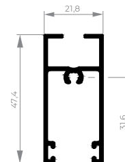
CEL-053 Travessa da folha 0,473 kg/m
