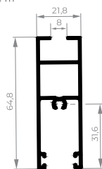
CEL-246 Travessa inferior da folha 0,686 kg/m
