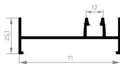
CEL-791 Marco lateral com contrafecho 0,500 kg/m
